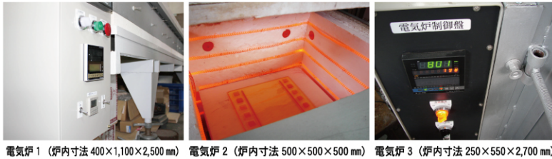
電気炉 1 (炉内寸法 400×1,100×2,500 mm) 電気炉 2 (炉内寸法 500×500×500 mm) 電気炉 3 (炉内寸法 250×550×2,700 mm)
